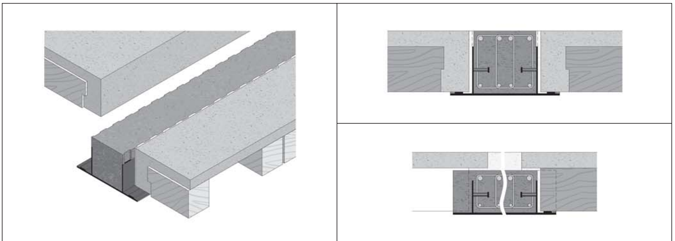
Stropy zespolone drewniano-betonowe (część betonowa prefabrykowana). Żebra drewniane.
