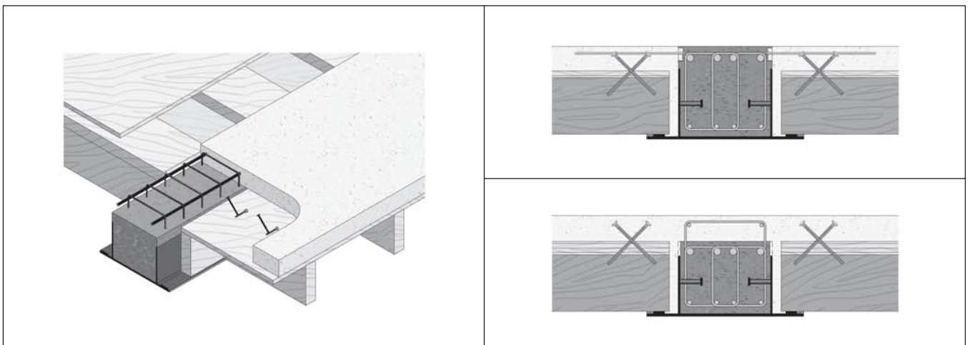
Stropy zespolone drewniano-betonowe (część betonowa wylewana na mokro). Żebra drewniane.
